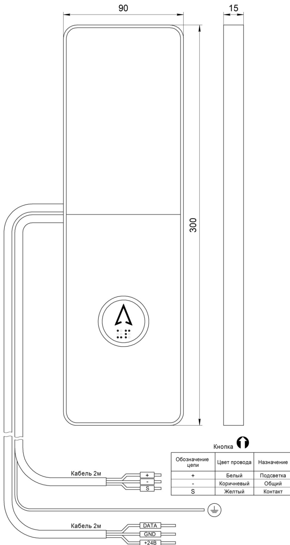
Рис.1 Внешний вид Вызывной пост ОНИКС НШЕК.468381.027
